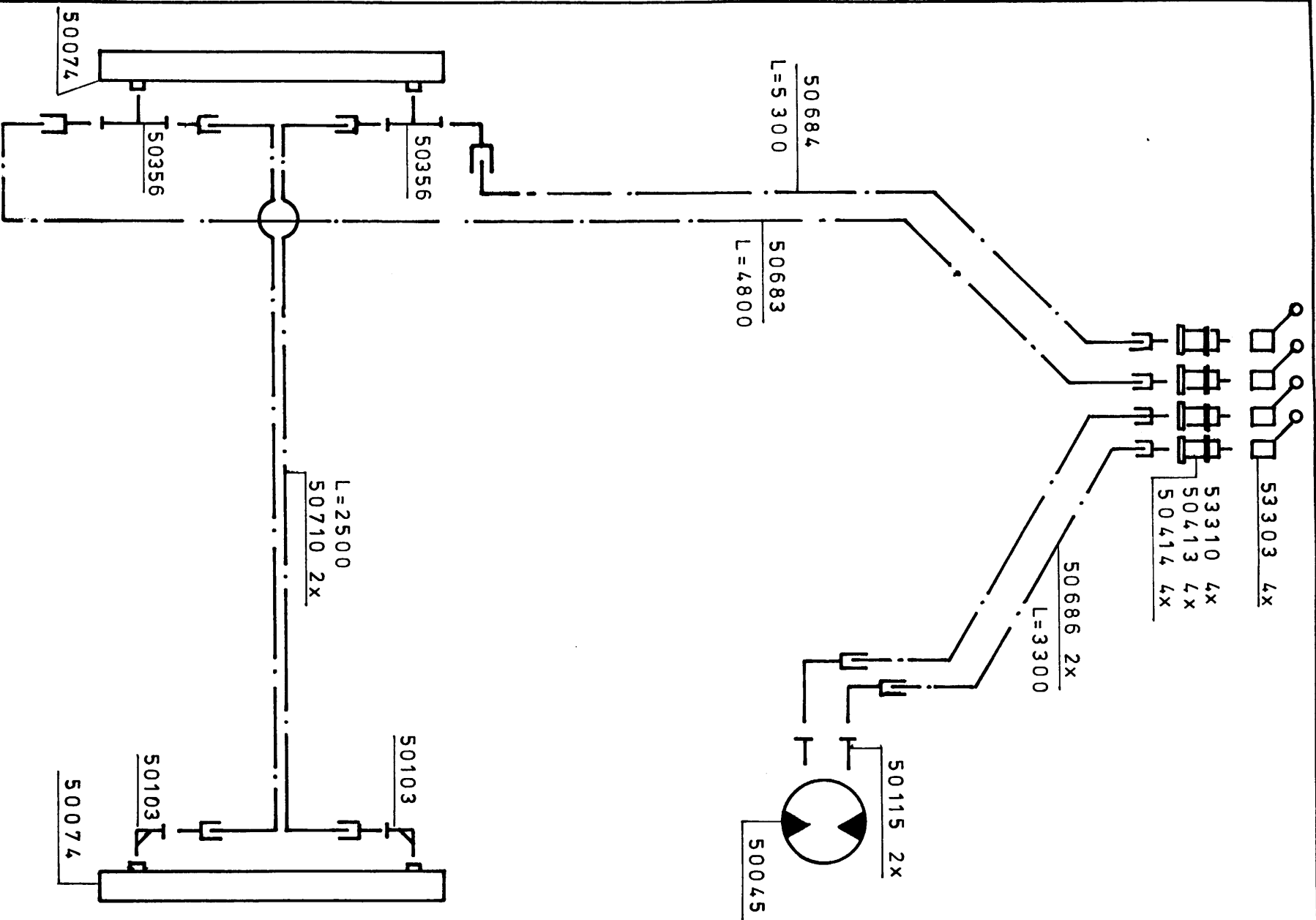
Afb. 1 Schema standaard hydrauliek Standard hydraulik Schema
