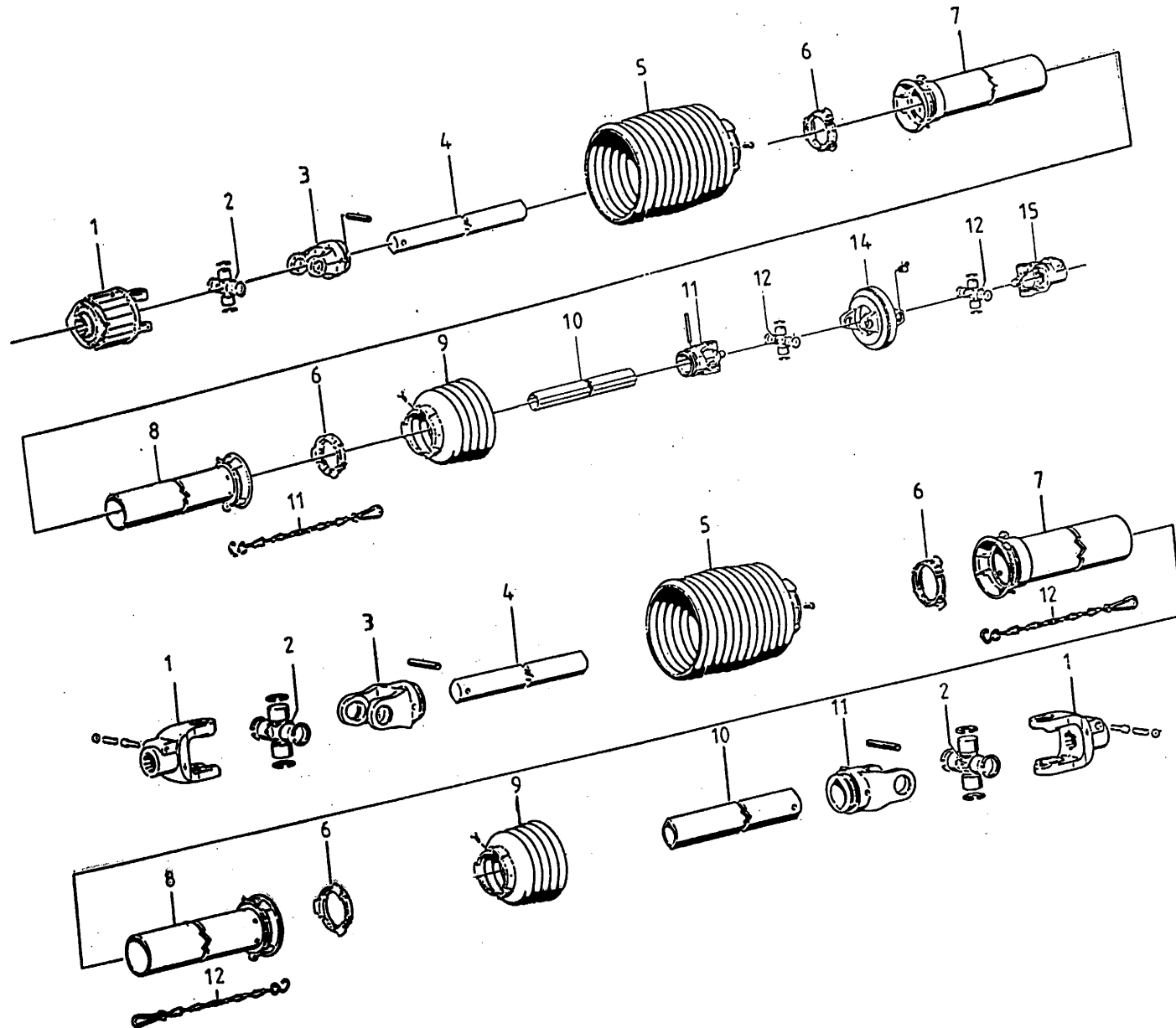
Afbeelding 18 Aftakassen Gelenkswellen
