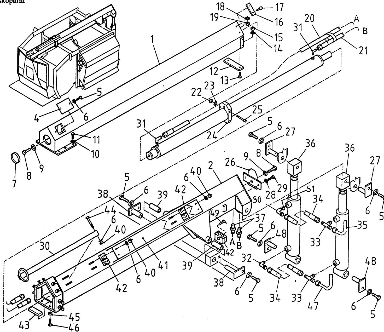
Afbeelding 7 Teleskoop Teleskoparm
