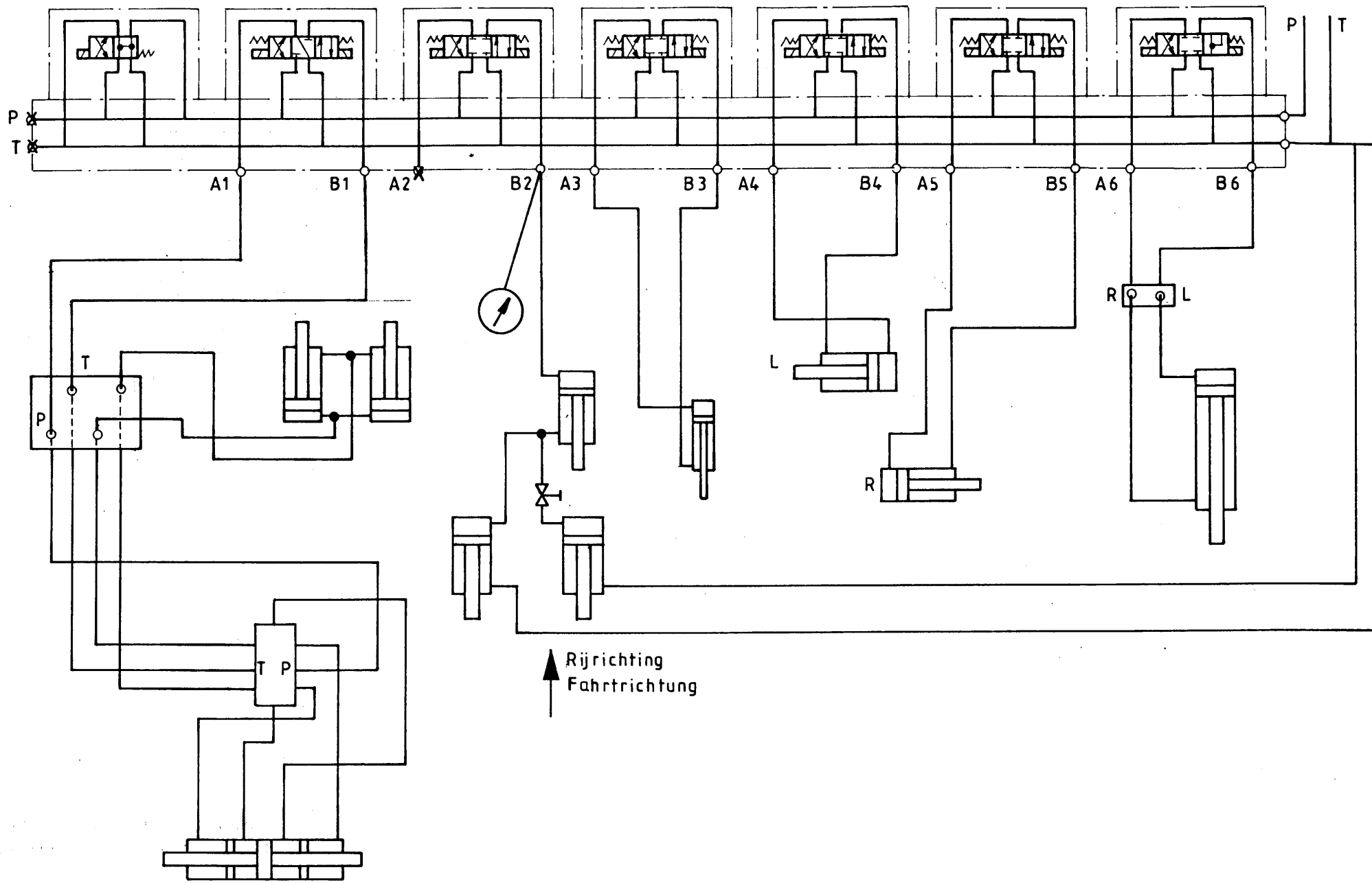
Abbeelding 21 Hydraulisch schema elektrische bediening Hydraulischer Schaltplan elektrische Fernbedienung
