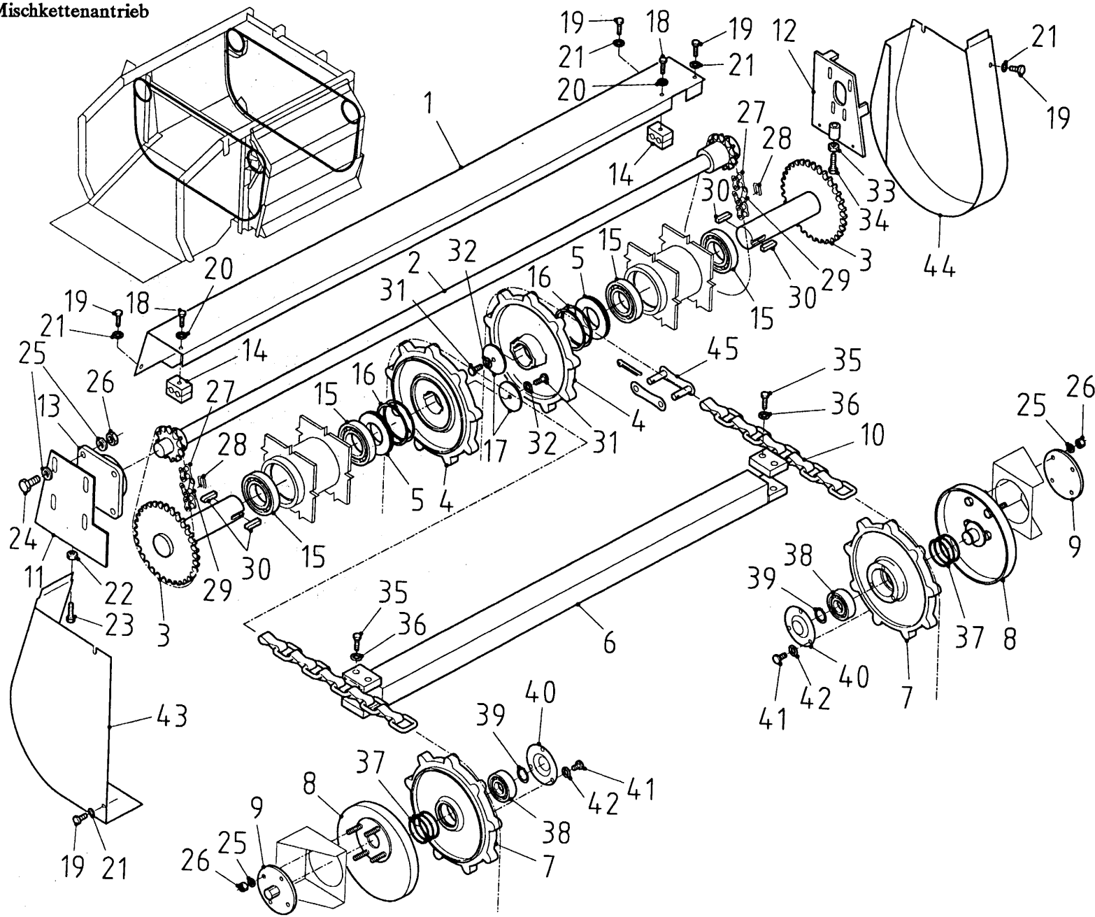
Afbeelding 4 Mengkettingaandrijving Mischkettenantrieb
