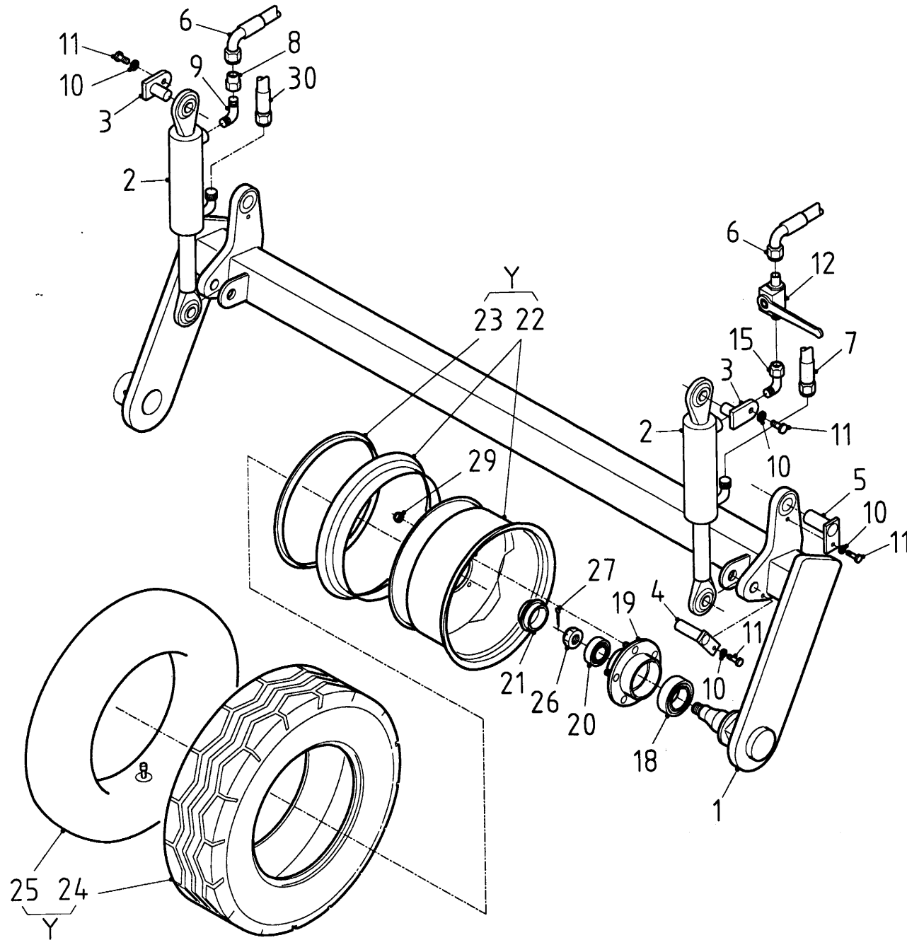
Afbeelding 3 Wielset Radachse
