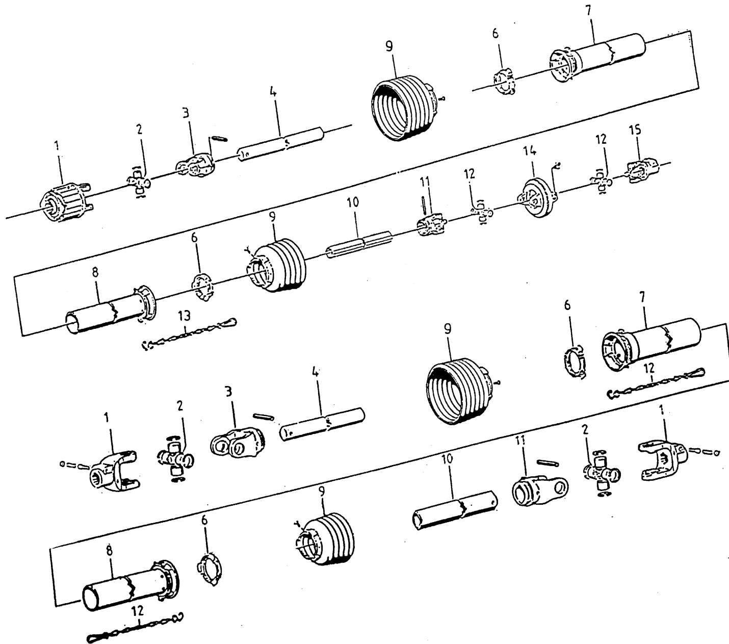
Afbeelding 18 Aftakassen Gelenkwellen
