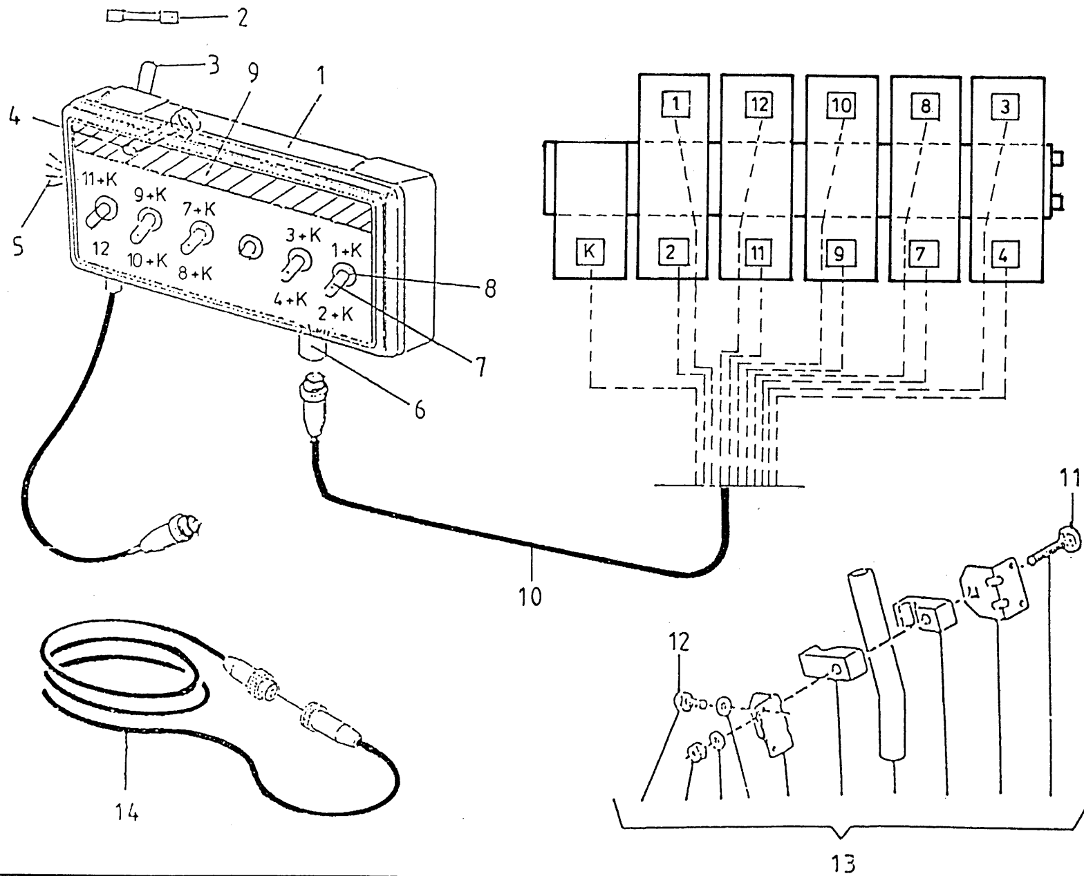
Afbeelding 14 Bedieningskast en aansluitschema Bedienungspult und Schaltplan
