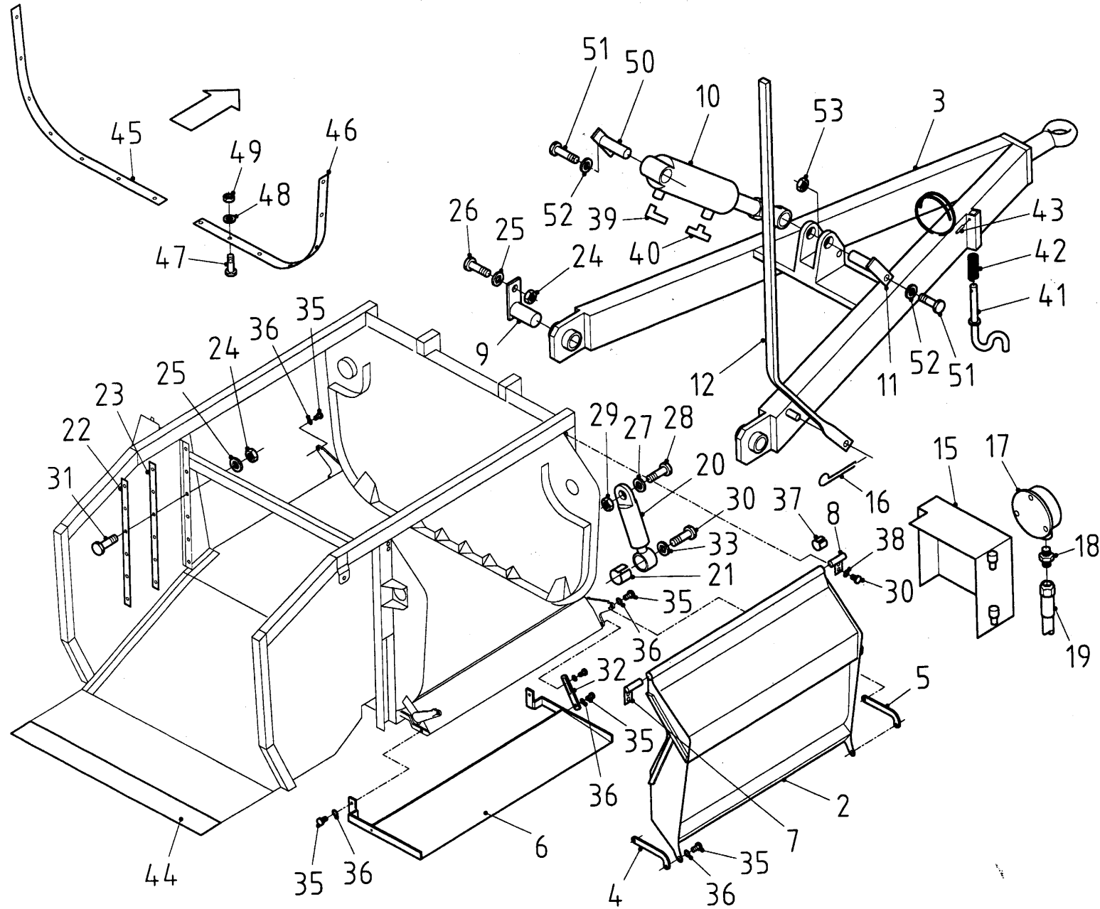
Afbeelding 2 Frame Rahmen
