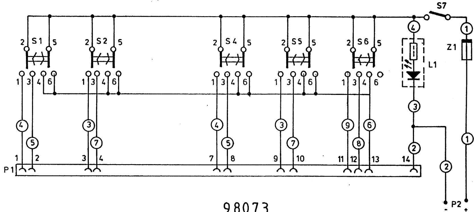
Afbeelding 22 Elektrisch schema Elektrischer Schaltplan
