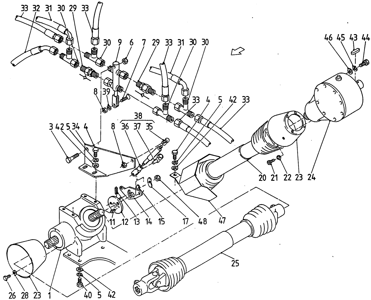
Afbeelding 5 Aandrijving Antrieb
