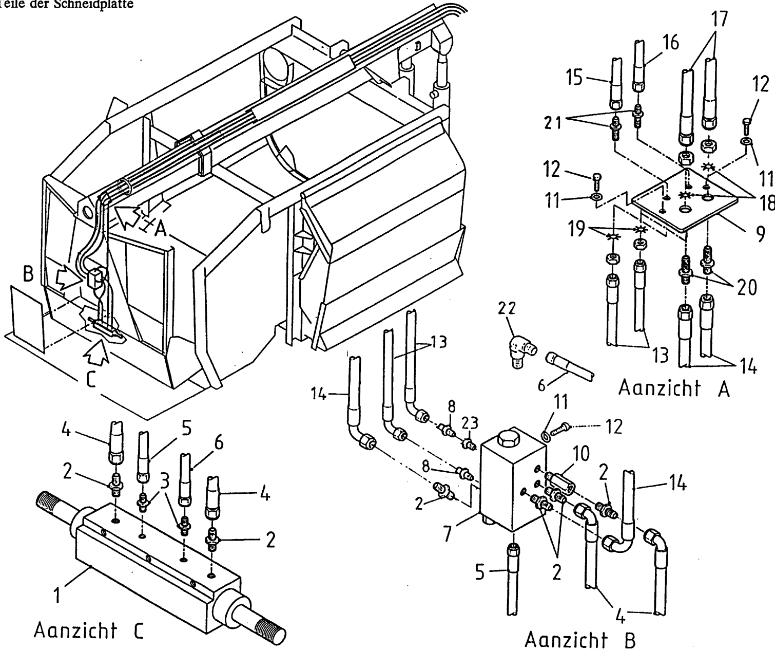
Afbeelding 9 Snijbordcomponenten Teile der Schneidplatte
