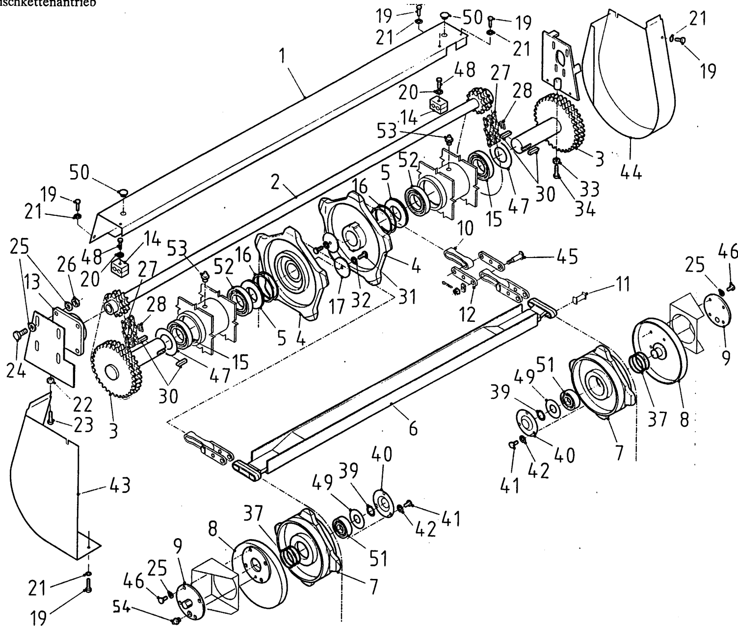
Afbeelding 4 Mengkettingaandrijving Mischkettenantrieb
