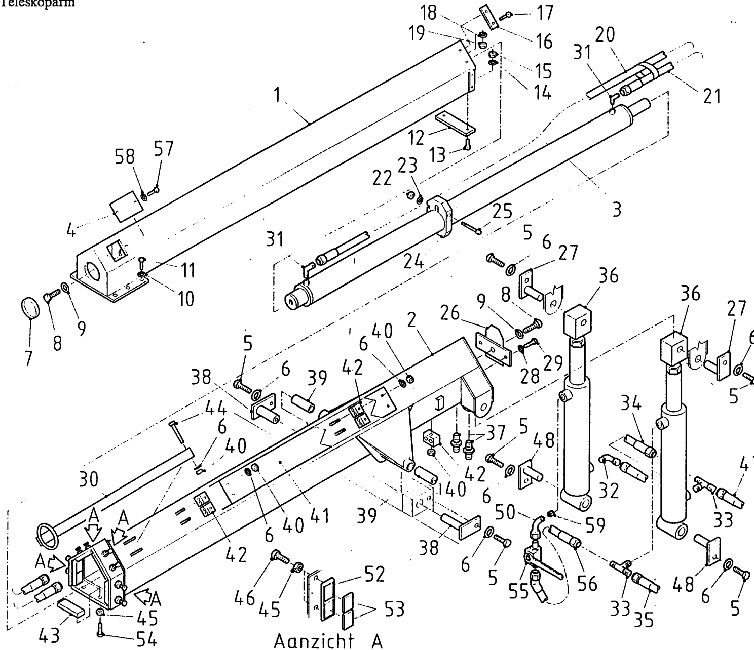
Afbeelding 7 Telescoop Teleskoparm
