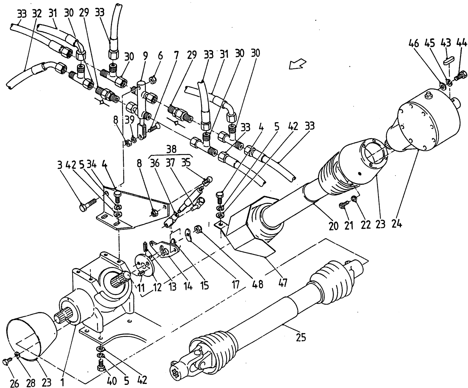
Afbeelding 5 Aandrijving Antrieb
