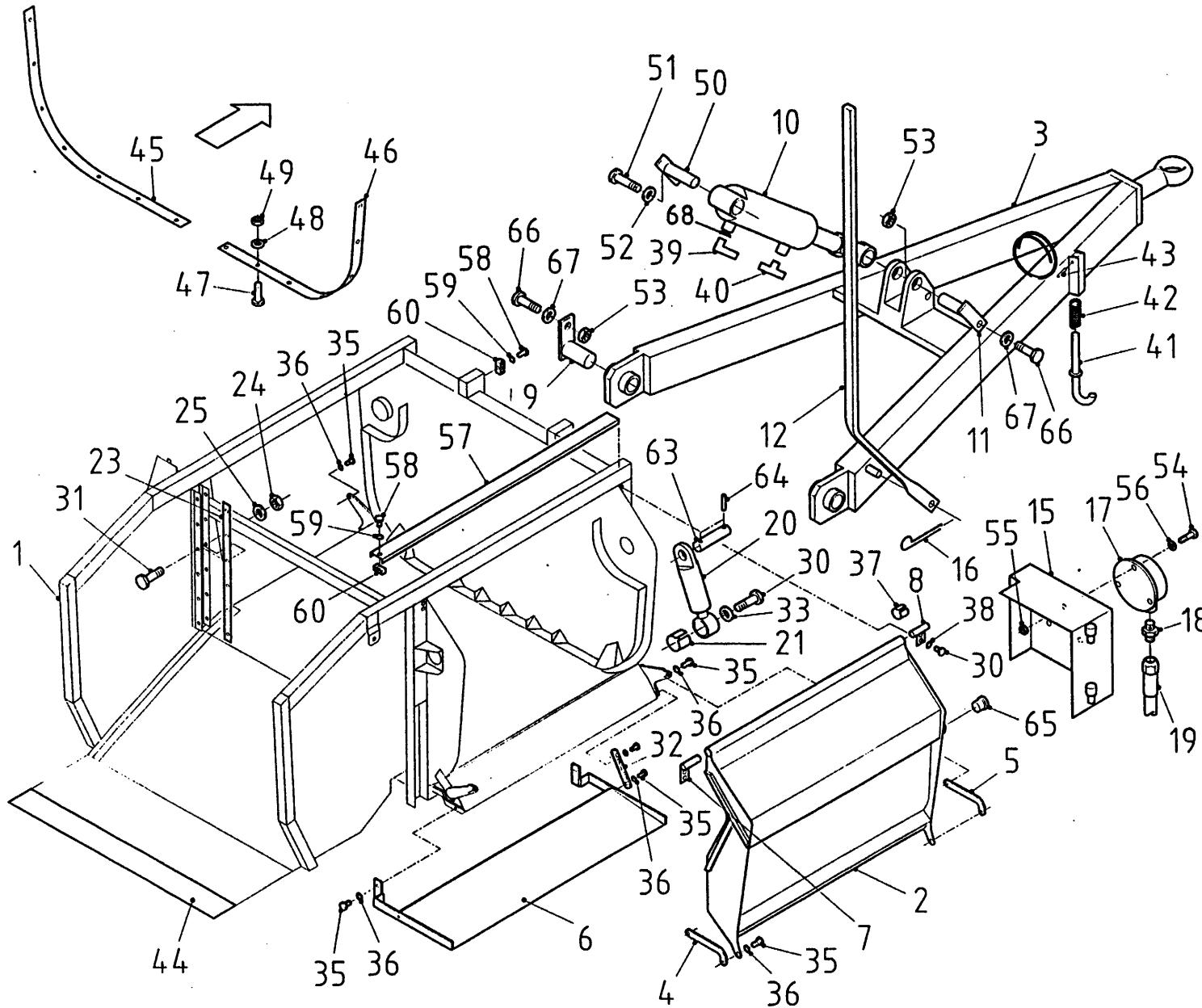
Afbeelding 2 Frame Rahmen
