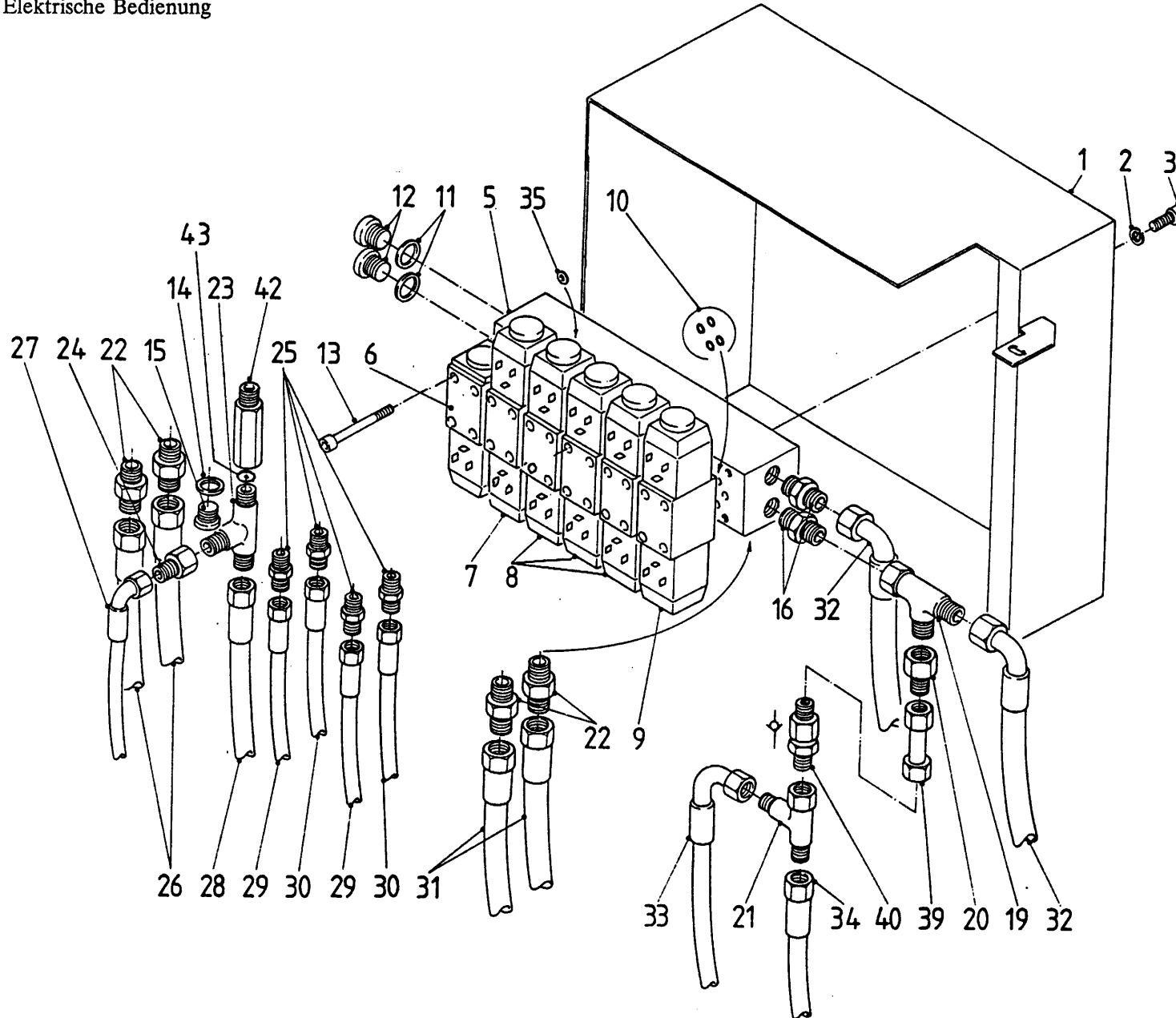
Afbeelding 13 Elektrische bediening Elektrische Bedienung
