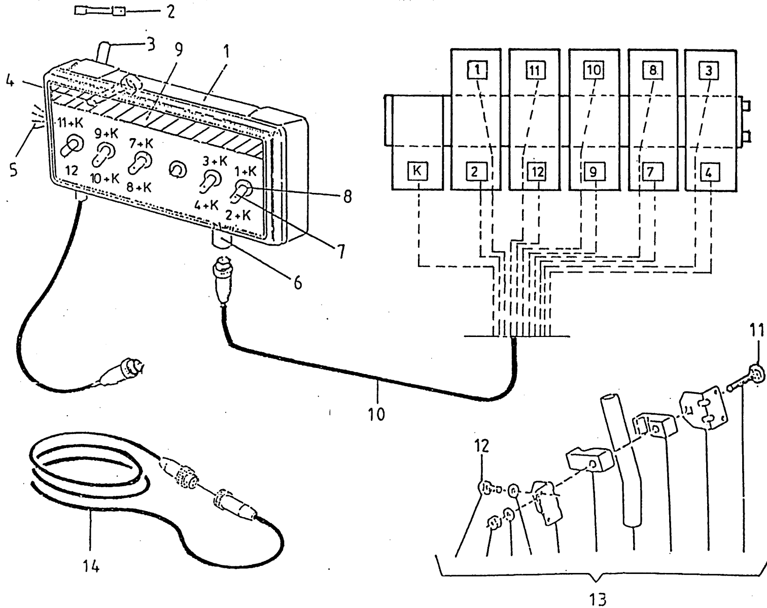
Afbeelding 14 Bedieningskast en aansluitschema Bedienungspult und Schaltplan
