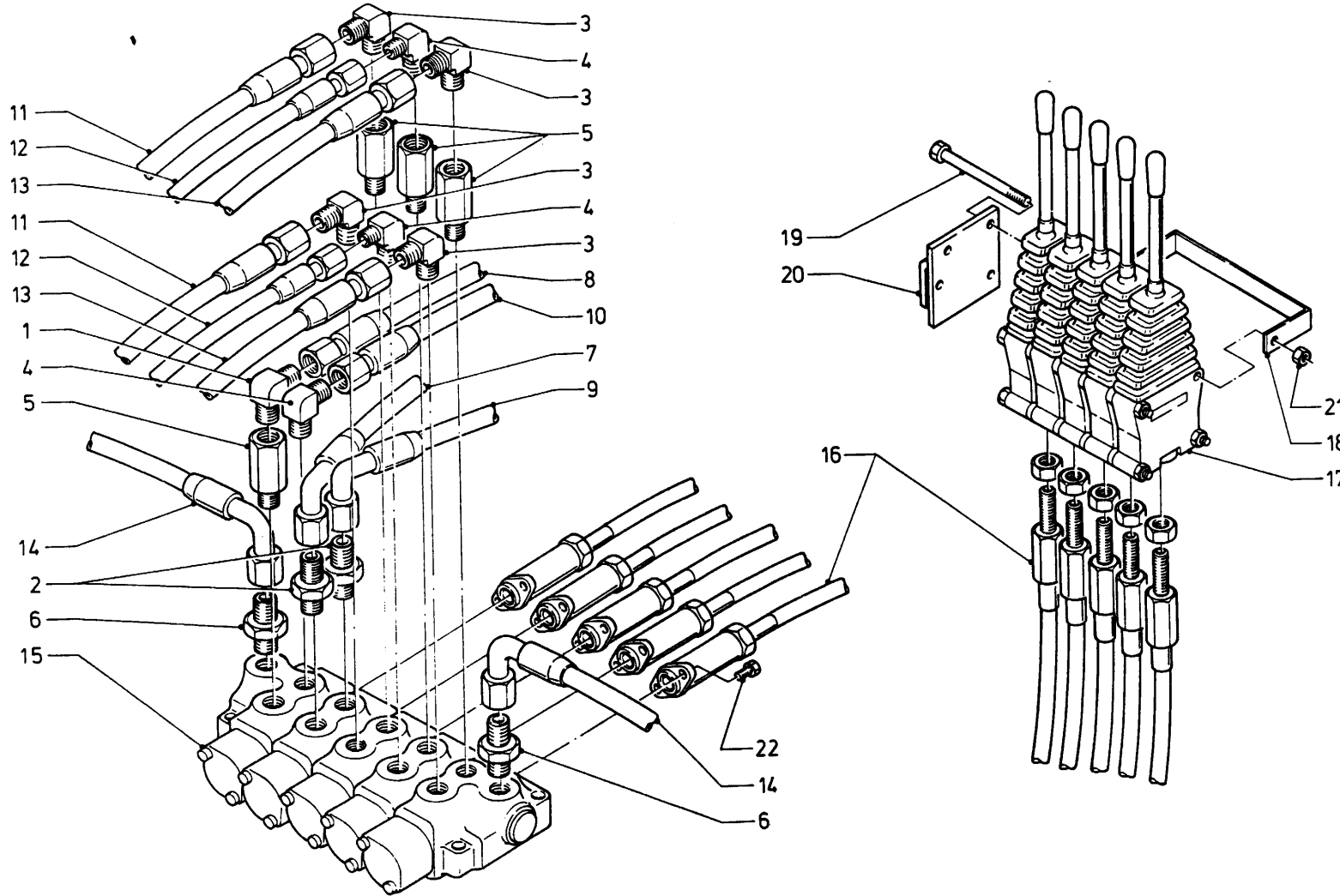
Afb. 9 Ventielblok en afstandsbediening Steuerblock und Fernbedienung Valves with remote control Valves avec commande à distance
