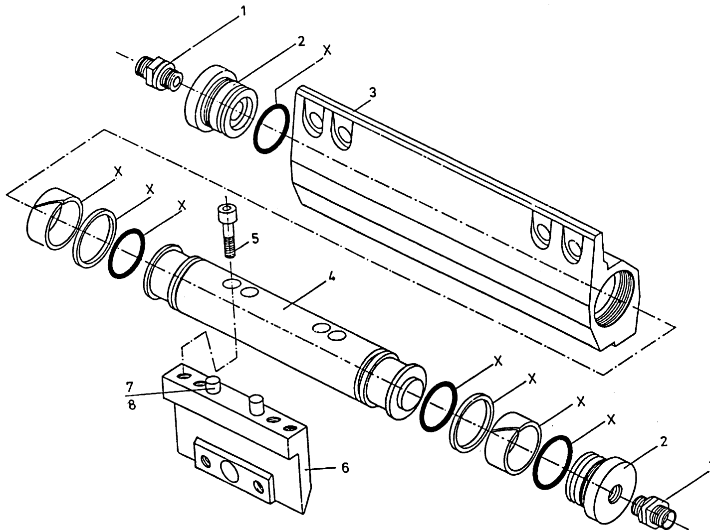
Afb. 6 Achtermescylinder 50055 Zylinder Hintermesser Main knife cylinder Vérin pour scie arrière
