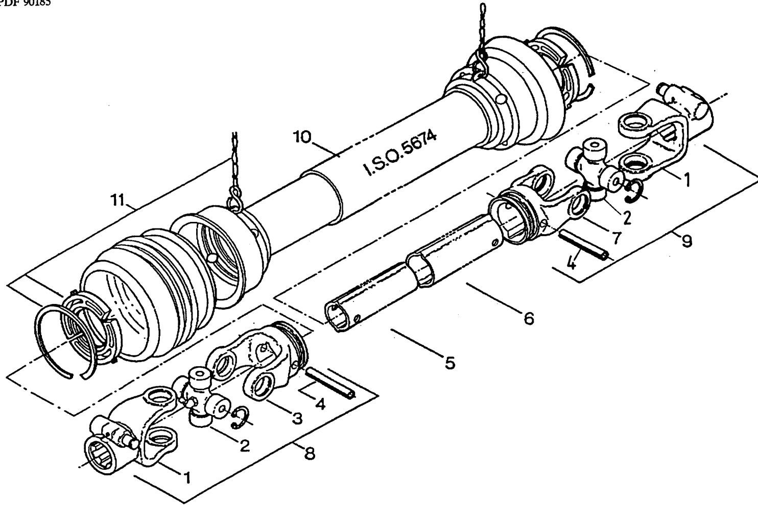
Abbeiding 3 Aftakas 90185 Zapfwelle 90185 PTO-shaft 90185 Arbre de PDF 90185
