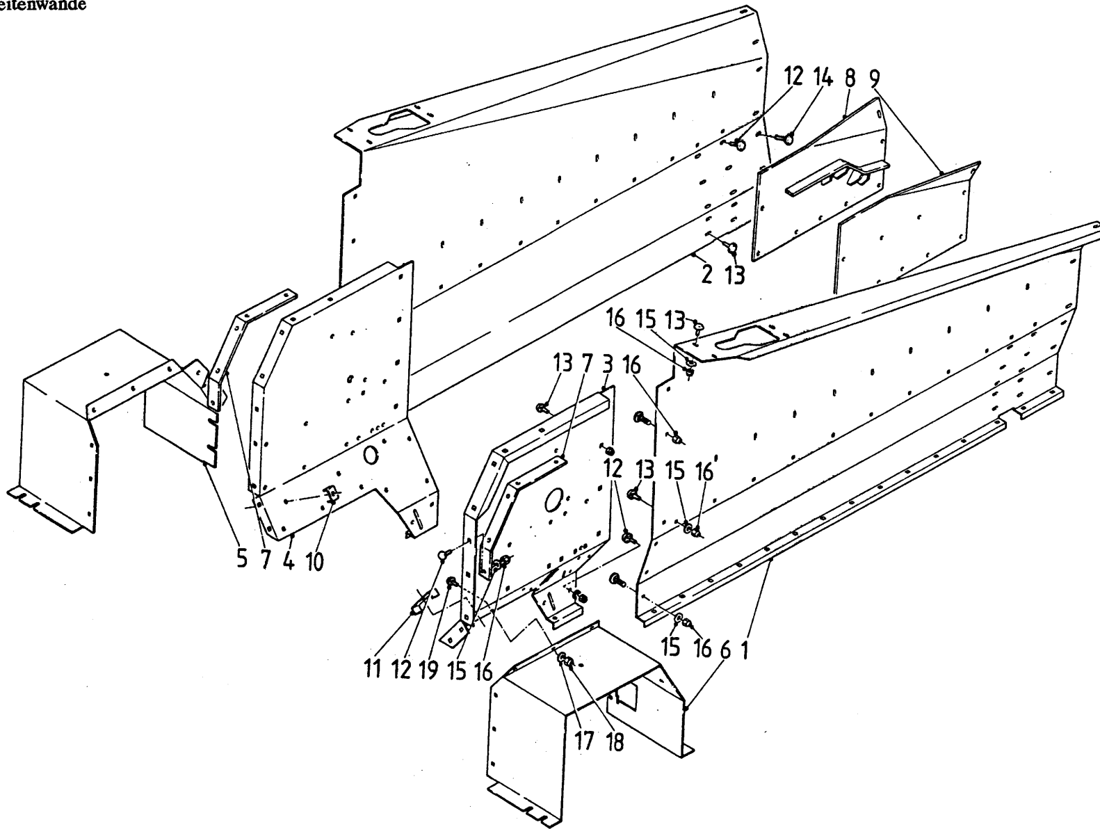
Afb. 3 Zijbeplating Seitenwände
