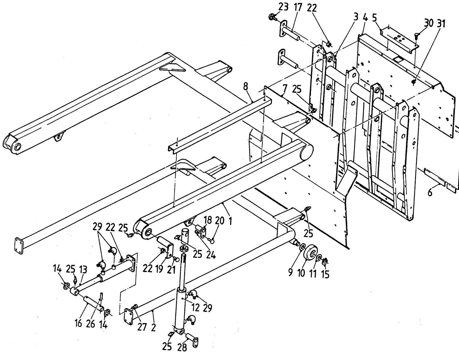
Afb. 10 Laadinrichting Laadsysteem
