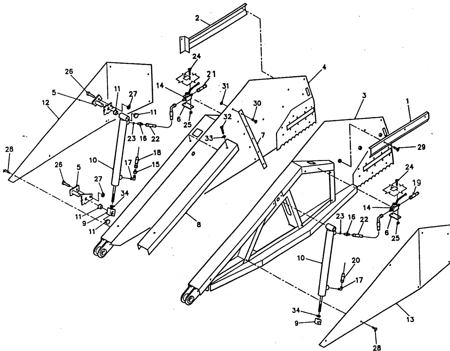
Afbeelding 11 Snijframe zijwanden Schneidschild Seitenwände
