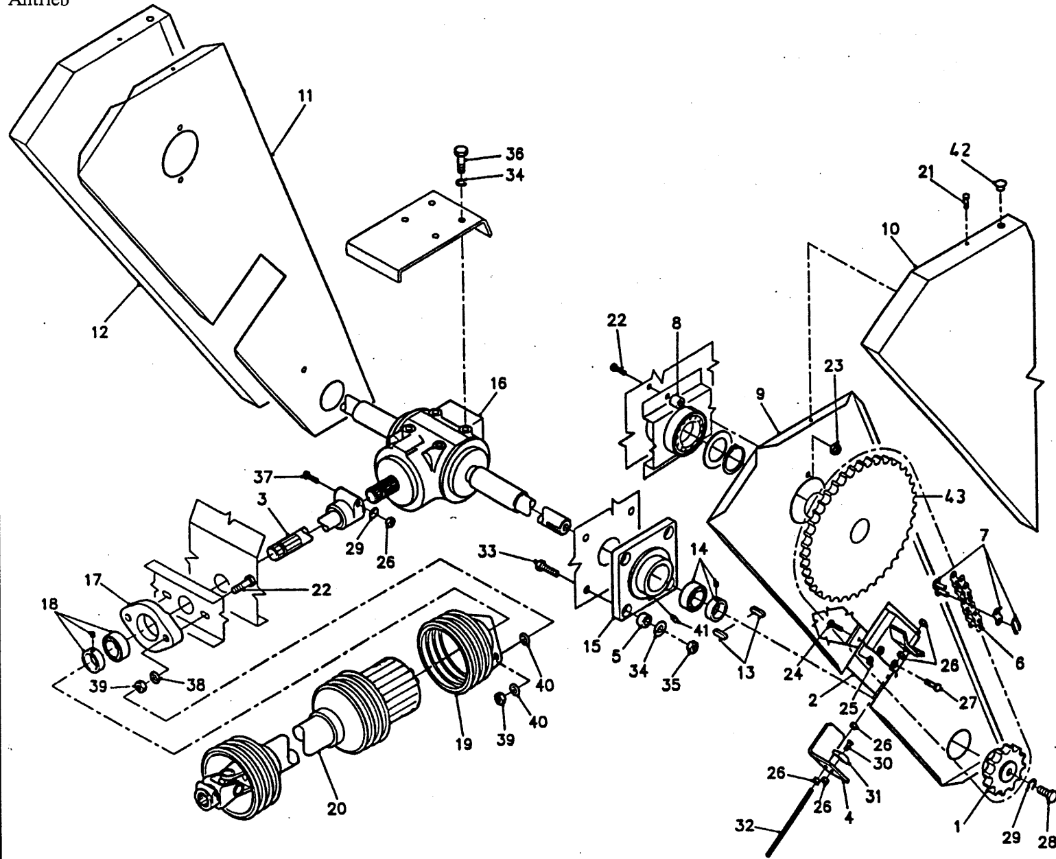
Abbeelding 7 Aandrijving Antrieb
