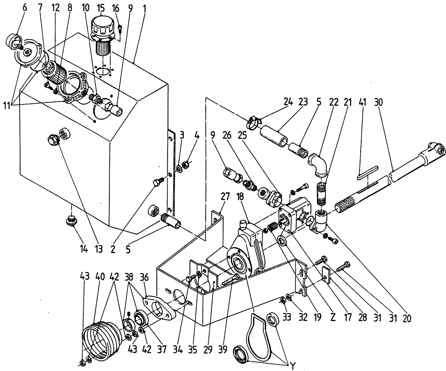
Afbeelding 21 Pompunit Pumpeneinheit
