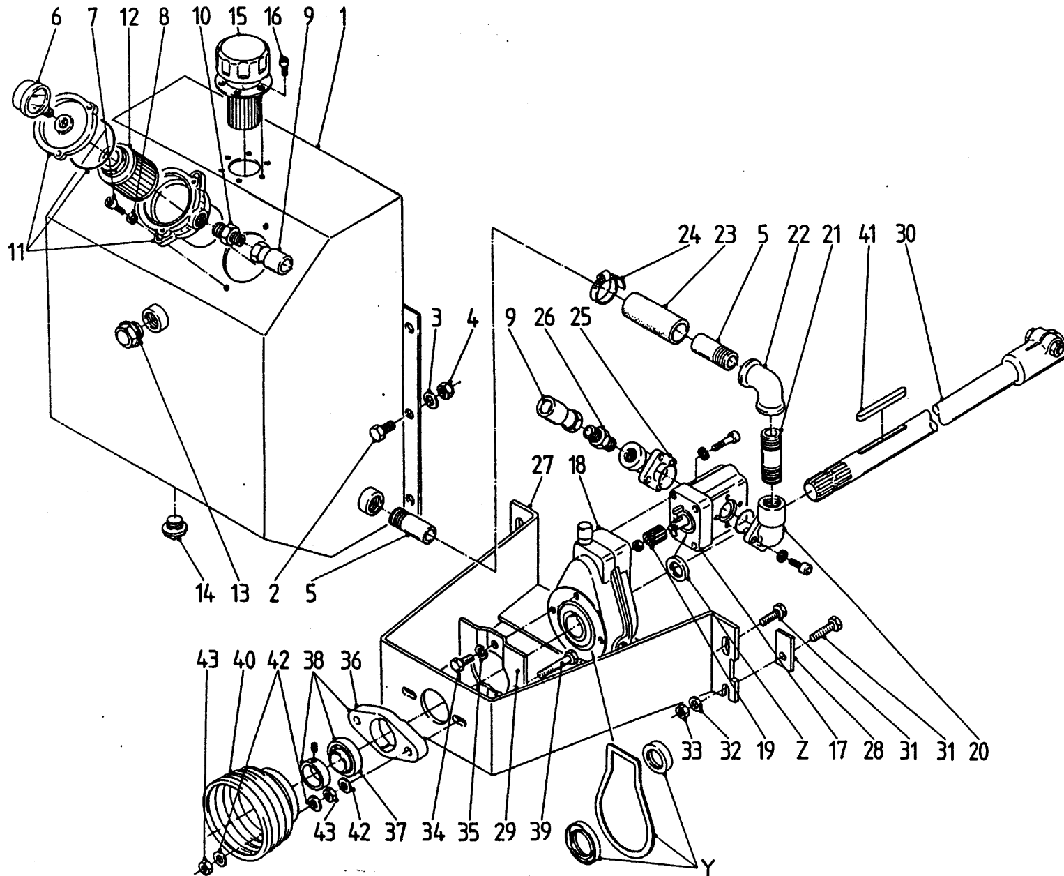
Afbeelding 21 Pompunit Pumpeneinheit
