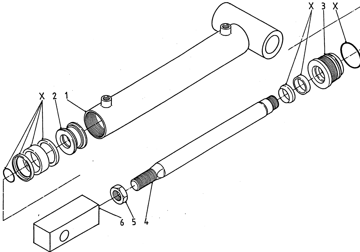
Afbeelding 19 Aanzetcilinder Vorschubcilinder
