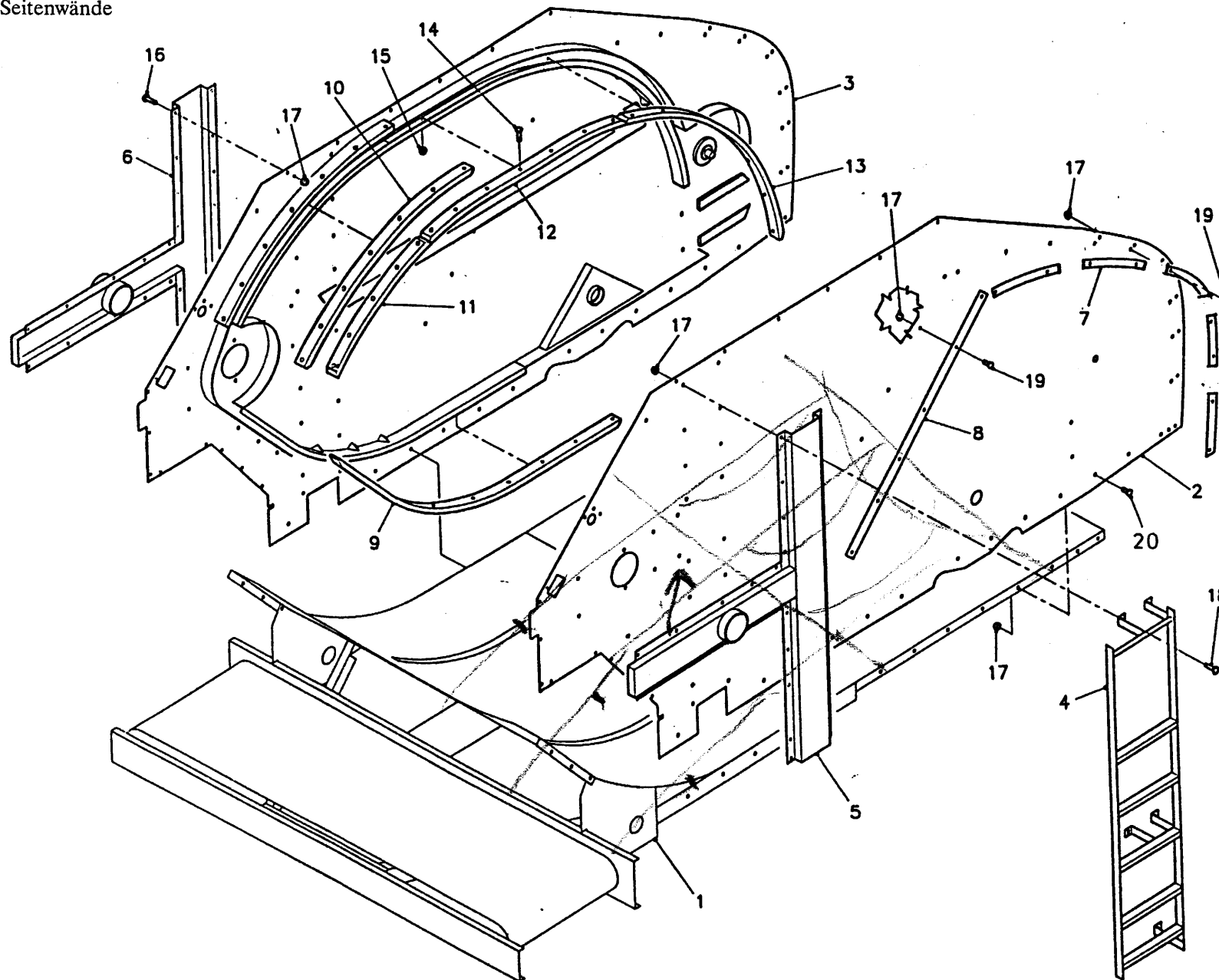
Afbeelding 4 Zijwanden Seitenwände
