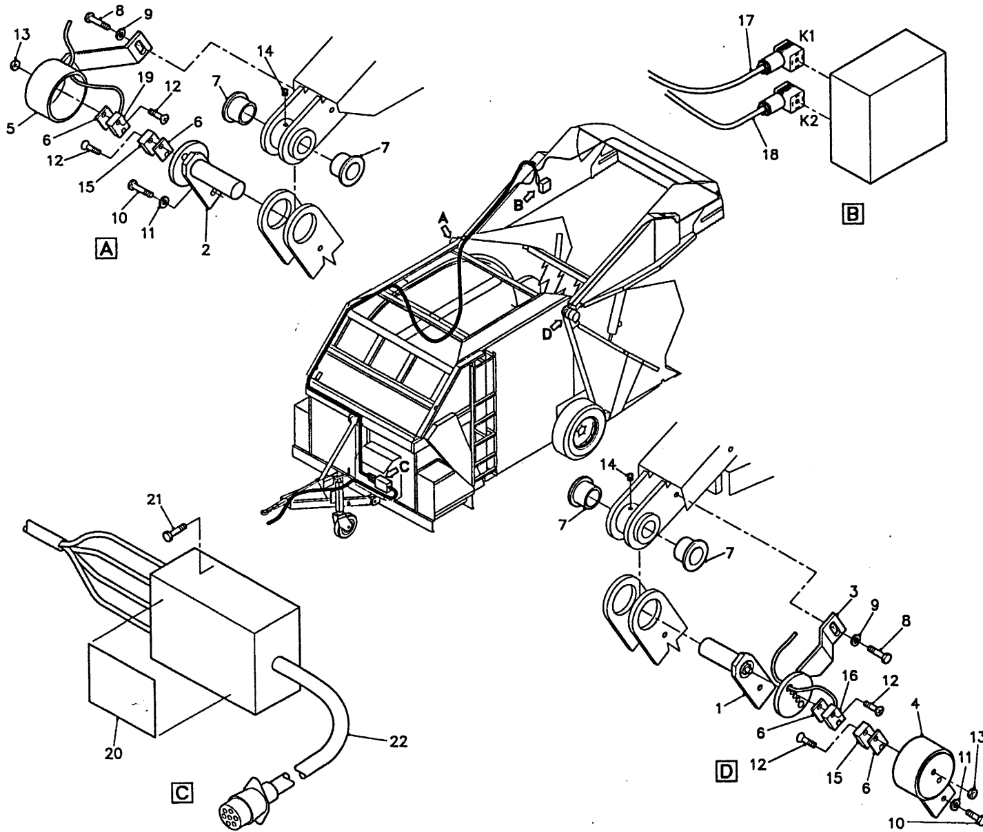
Afbeelding 14 Gelijkloopsysteem Ausgleichssystem
