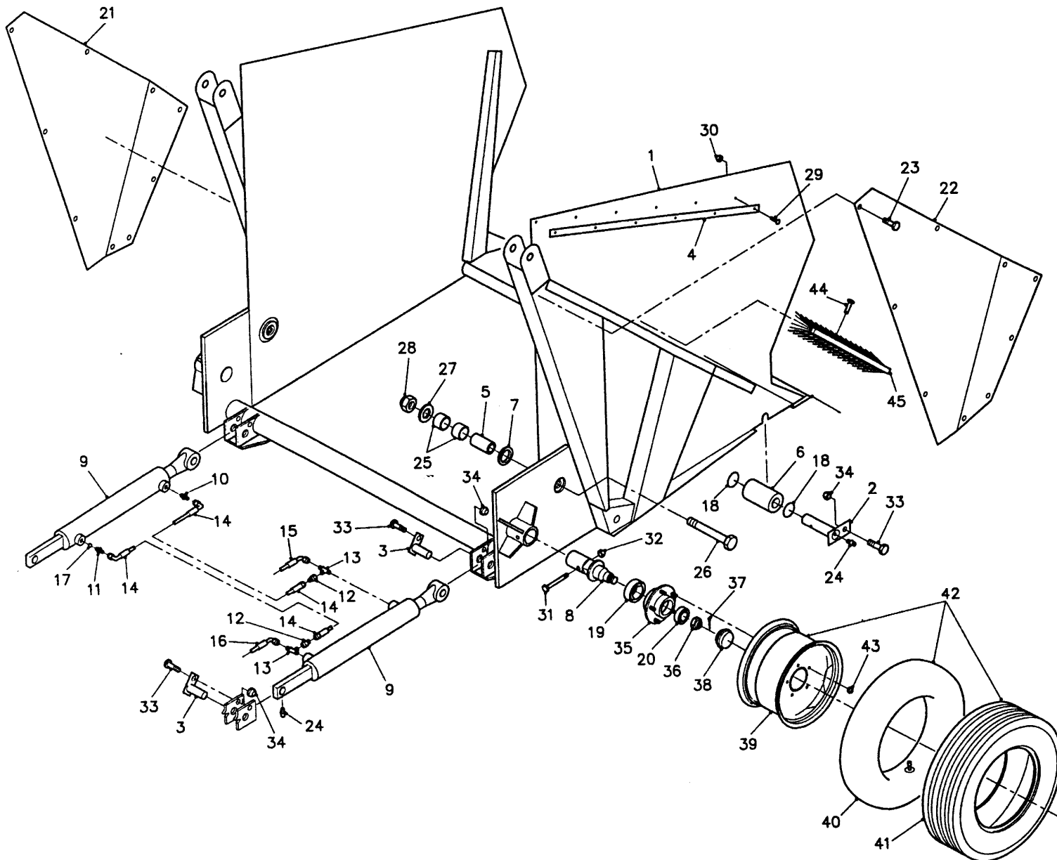
Afbeelding 10 Laadklep Ladeklappe
