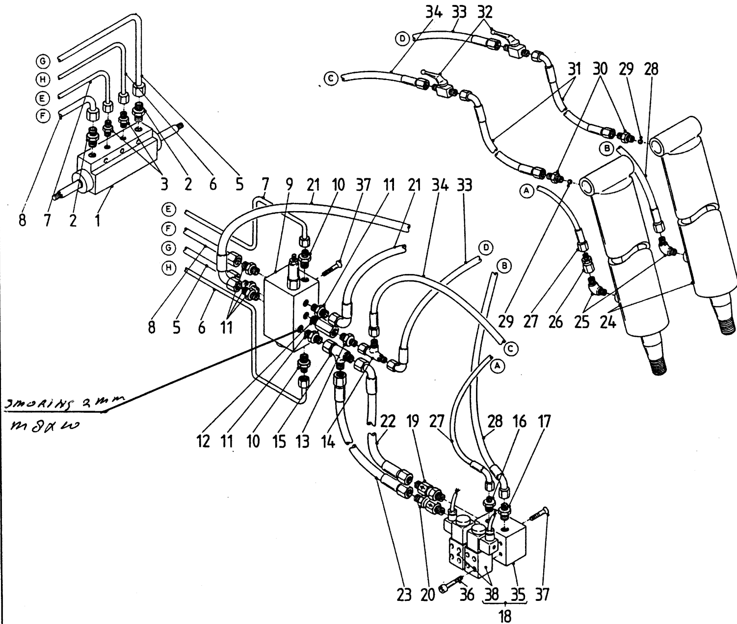
Afbeelding 13 Schakelblok + gelijkloopventiel Schaltblock + Gleichlaufventil
