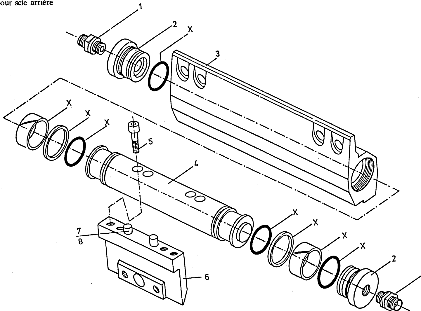
Afb. 6 Achtermescilinder Zylinder Hntermesser Back knife cylinder Vérin pour scie arrière
