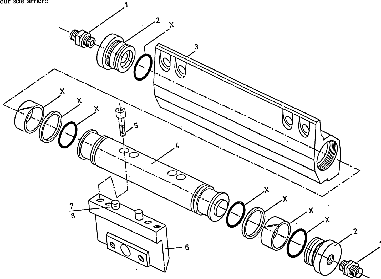
Afb. 6 Achtermescylinder Zylinder Hntermesser Back knife cylinder Vérin pour scie arrière
