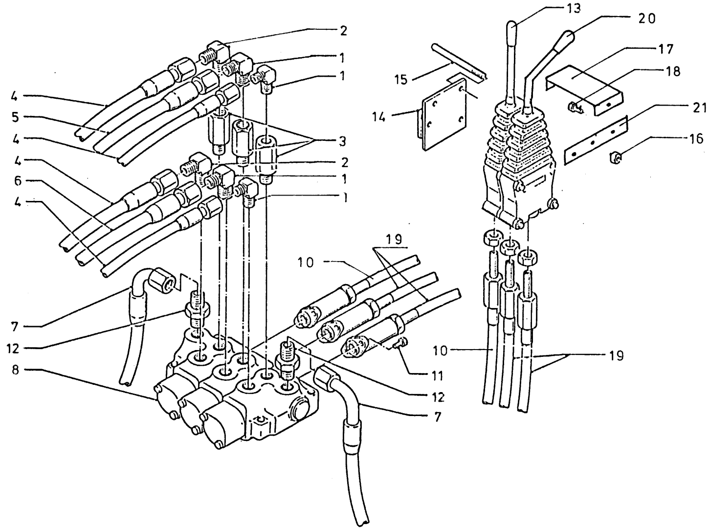
Afb. 10 Ventielblok en afstandsbediening Steuerblock und Fernbedienung Valves with remote control Valves avec commande à distance
