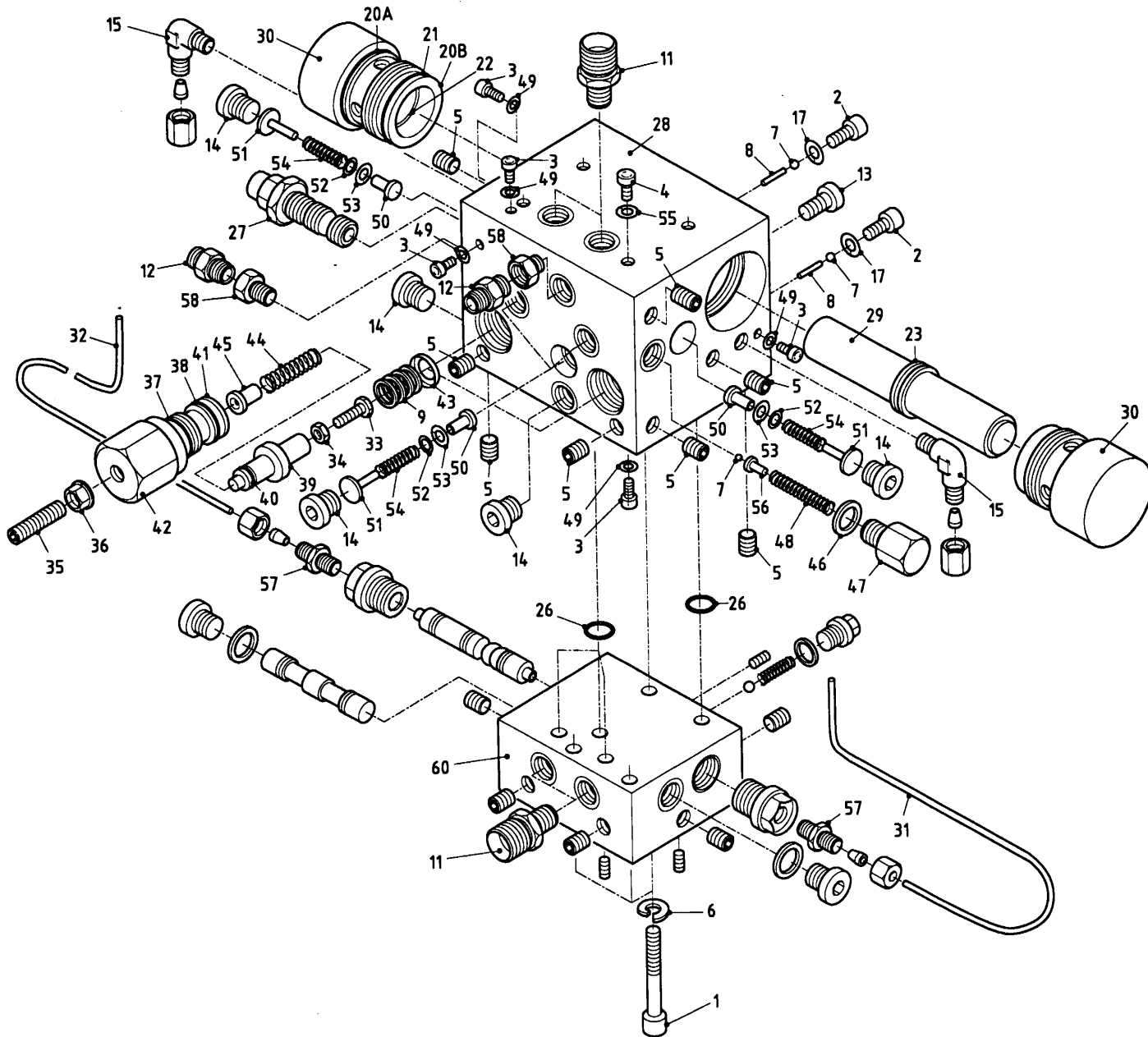
Afb. 7 Stuurblok inwendig Steuerventil innenseite
