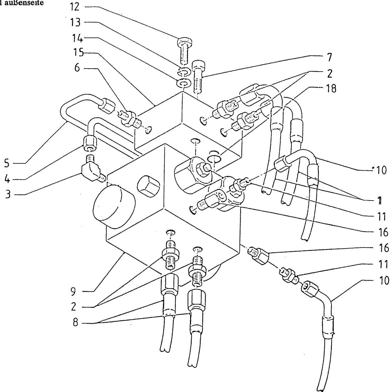
Afb. 6 Stuurblok uitwendig Stuervertil außenseite
