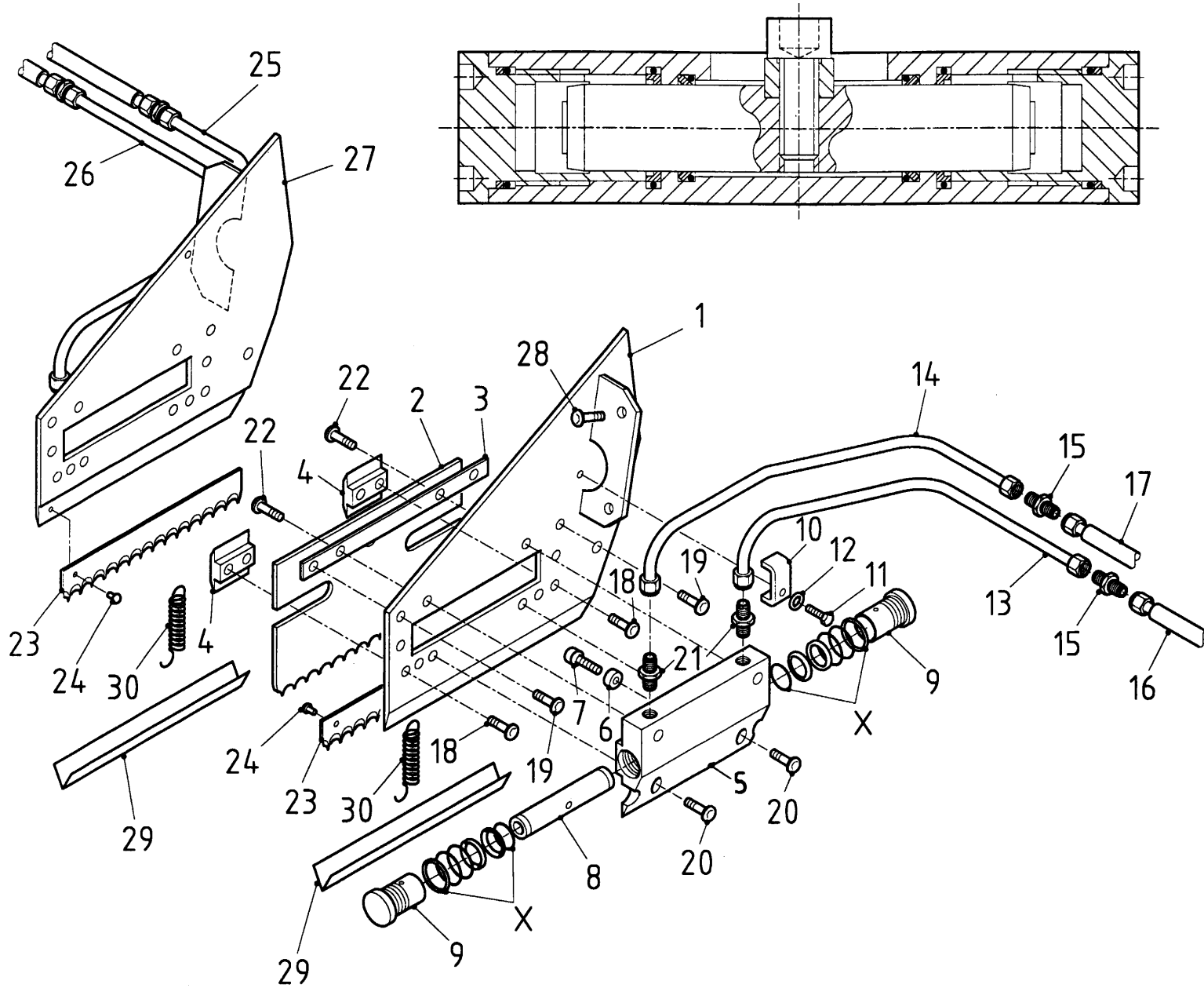
Afb. 5 Zijmessen Seitenmesser
