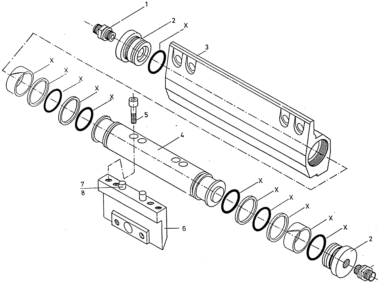
Afb. 10 Achtermescylinder Zylinder Hintermesser
